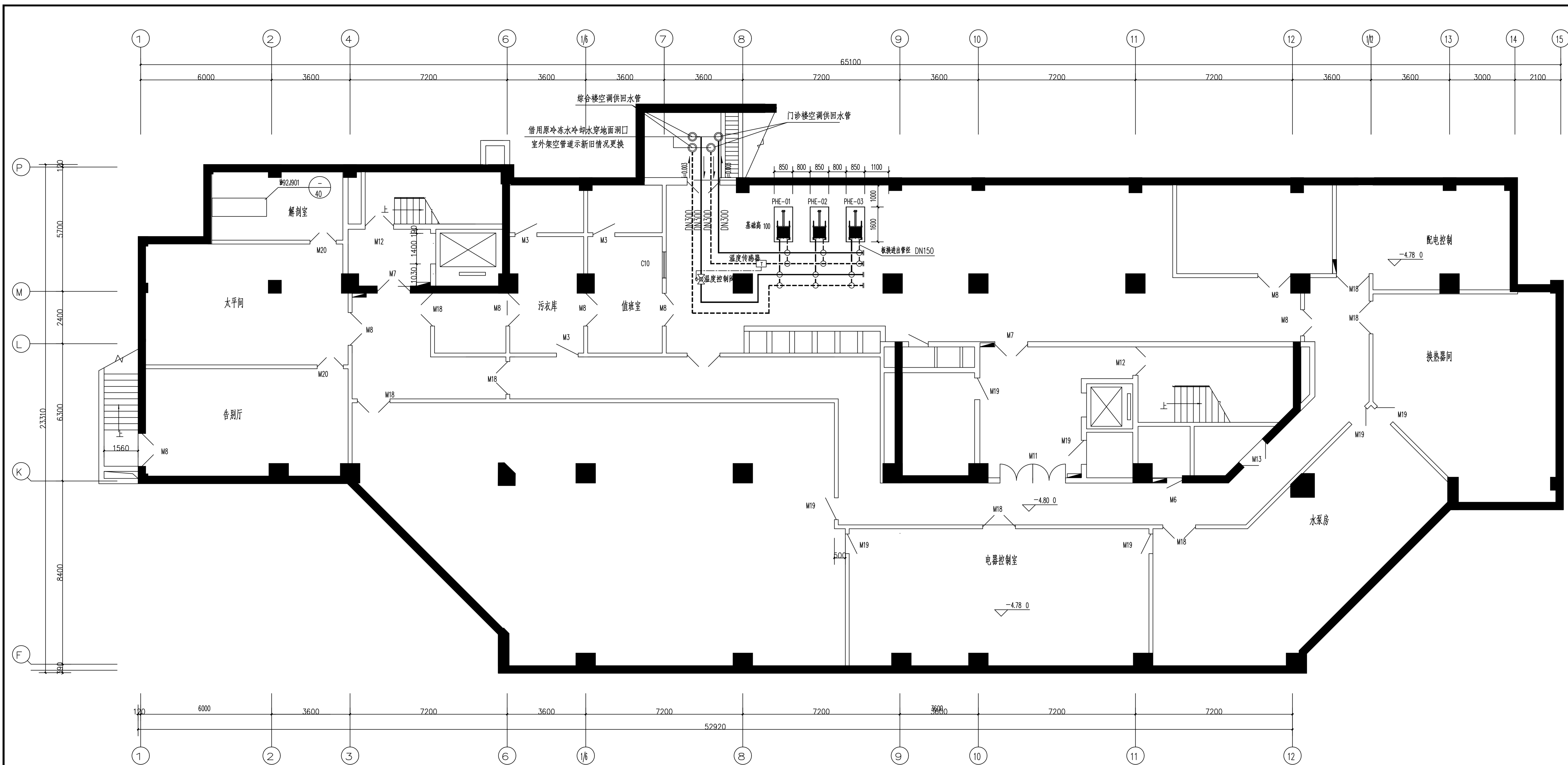
综合外科大楼地下一层空调干管平面图 1:100
